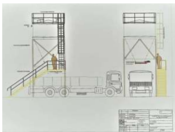
TOLVA DE FANGO PARA EDAR
